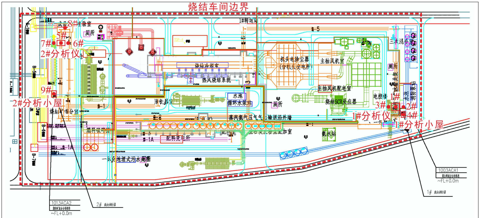
图 8-1 本项目辐射工作场所及周边背景值监测点位示意图
